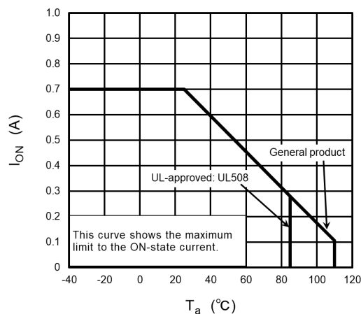
Fig. 14.1.2 I_{ON} - T_a
